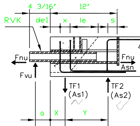
END ELEVATION
